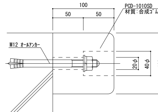
■PCD-1010SD 断面図
