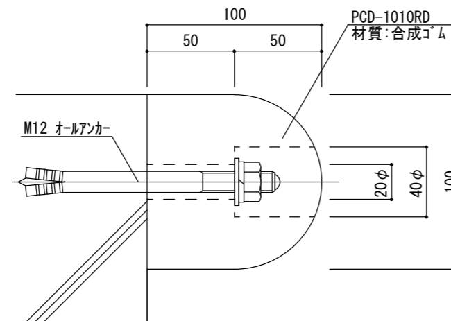
■PCD-1010RD 断面図
